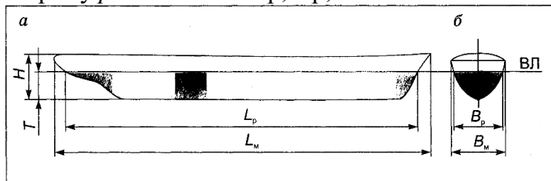
Рисунок 7 Главные размеры модели судна: а - главный вид; б - вид слева: L_p , B_p - расчётные длина и ширина; L_m , B_m - максимальная длина и ширина; H - высота борта; T - осадка; ВЛ – ватерлиния
