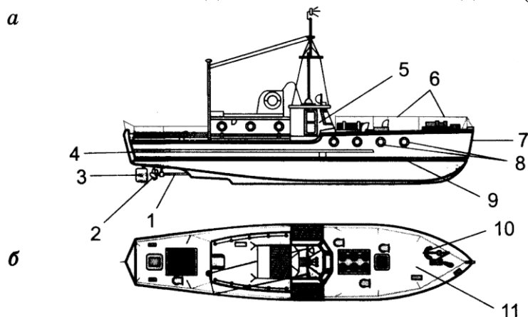
Рисунок 2 Управляемая модель катера фигурного курса с электродвигателем:
