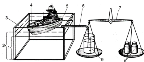
Рисунок 4 Определение водоизмещения судомодели опытным путём:
